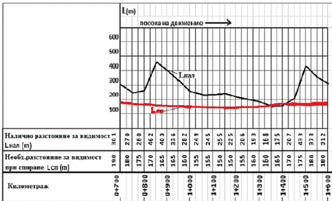
Фигура 9.1. Пример за анализ на видимостта при спирание
