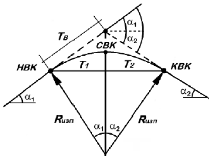
Фигура 6.2. Схема на изпъкнала вертикална крива
