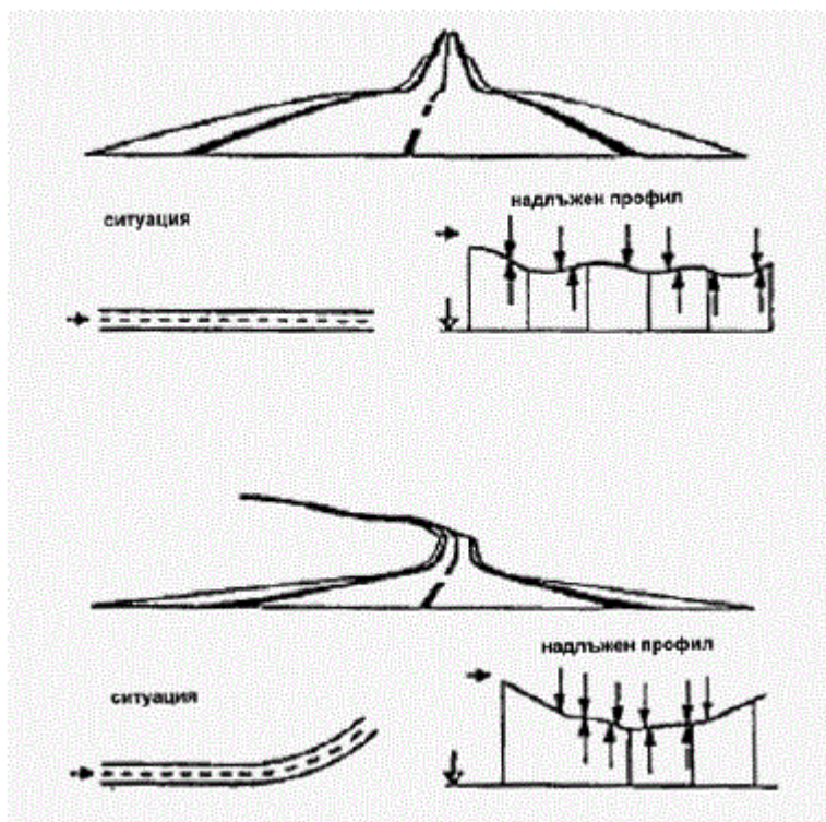
Фигура 22. Оптическо издуване
