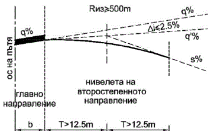
Фигура 46. Присъединяване на второстепенното към главното направление в
