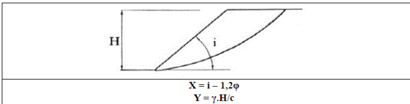
Фигура 102. Дрениран откос без опънна пукнатина
