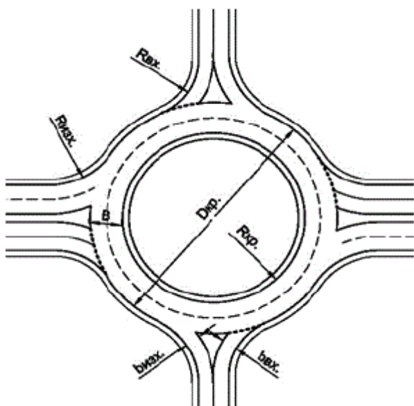
Фигура 50. Кръстовища от IV тип (кръгови кръстовища)
