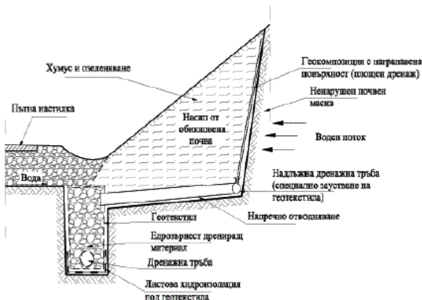
Фигура 131. Плочен дренаж под голям наклон, комбиниран с отвеждане на водата в подкопен дренаж с геотекстил
