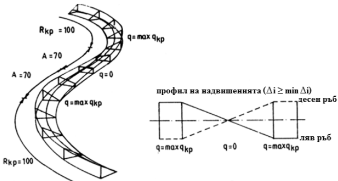
Фигура 8.1. Къса отсечка на преоформяне
