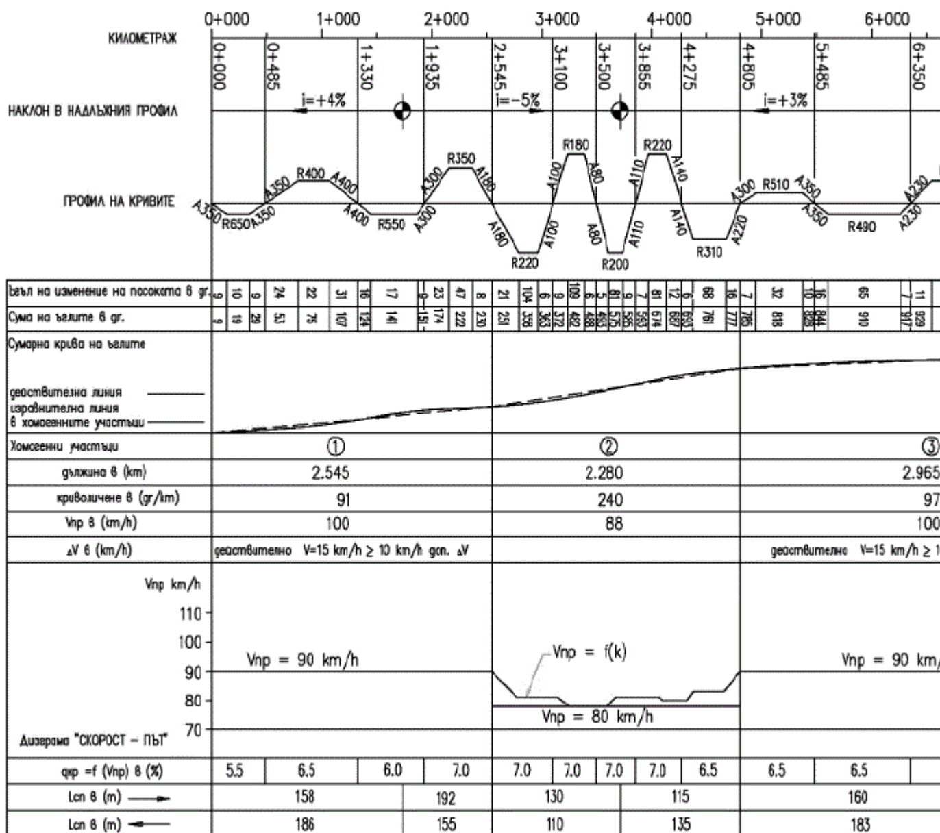
Фигура 1.6. Примерна диаграма "скорост - път" при обследване на съществуващ път
