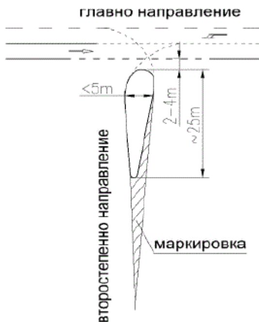
Фигура 58. Капковиден остров за кръстовища I тип
