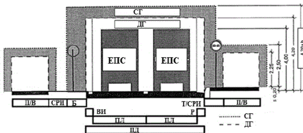
Фигура 31. Пътни габарити
