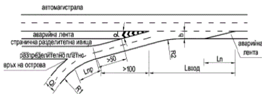
Фигура 94. Вход при директна и индиректна връзка
