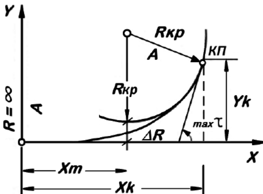
Фигура 4.2. Геометрия на клотоидата
