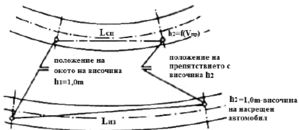
Фигура 9.3. Схематично положение на окото и на целевата точка (препятствието) при анализирането на разстоянията L_{\text{сп}} и L_{\text{из}}
