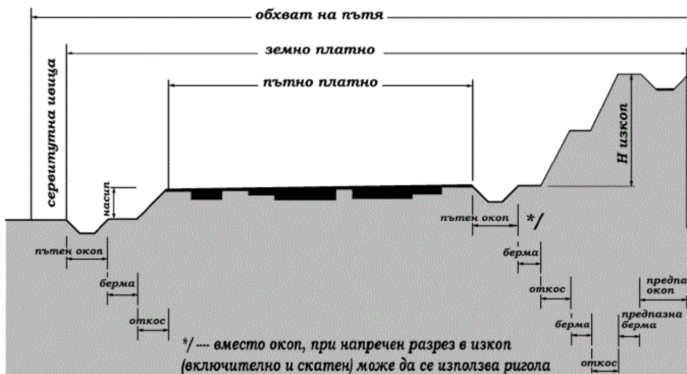
Фигура 29. Схематичен напречен профил
