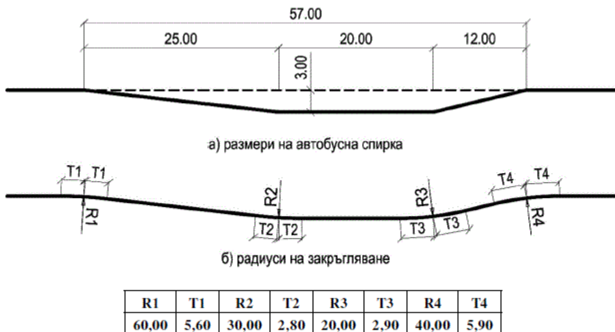
Фигура 40. Размери и радиуси на закръгление за автобусна спирка
