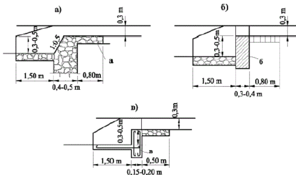
Фигура 112. Прагове в окопи ( i > 5\% ):
