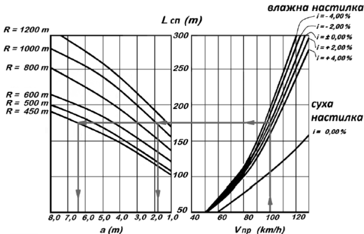
Фигура 10.3. Номограма за отчитане на L_{\text{сп}} и a^H за проверка на страничното разстояние за видимост
