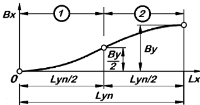
Фигура 7.1. Оформяне ръба на настилка при разширение на платното за движение
