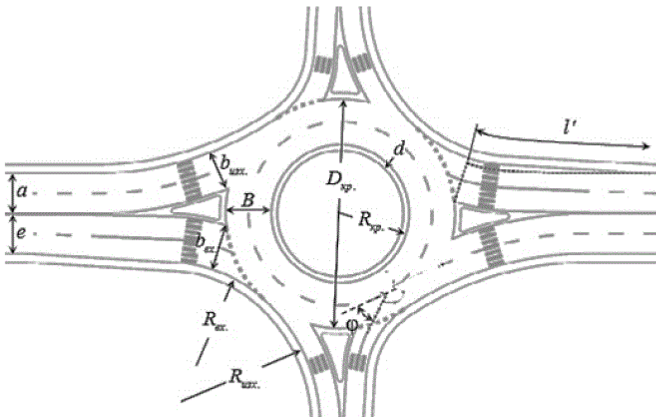
Фигура 64. Геометрични елементи на кръгово кръстовище
