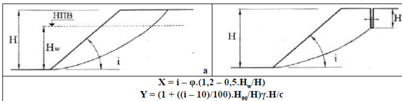
Фигура 101. Недрениран откос: а - обща схема; б - с опънна пукнатина
