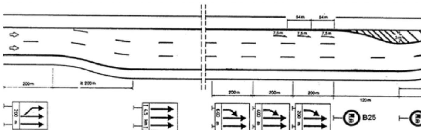
Фигура 12.1. Разположение и примерна сигнализация на допълнителна лента при нови автомагистрала с разширяване на платното от страна на средната разделителна ивица
