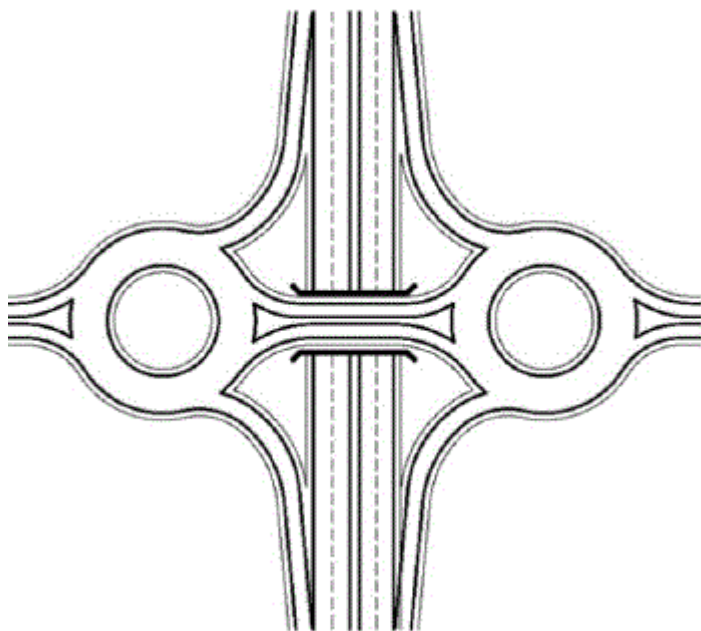
Фигура 62. Кръгово кръстовище с две съоръжения
