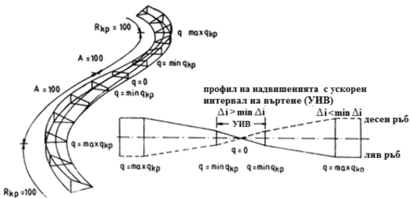
Фигура 8.2. Дълга отсечка на преоформяне
