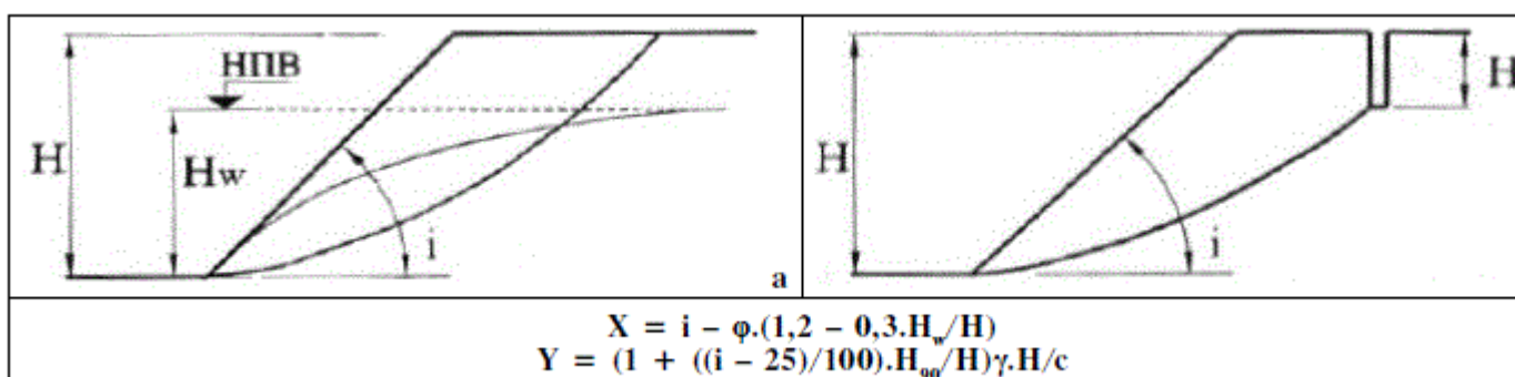
Фигура 100. Частично дрениран откос: а - обща схема; б - с опънна пукнатина
