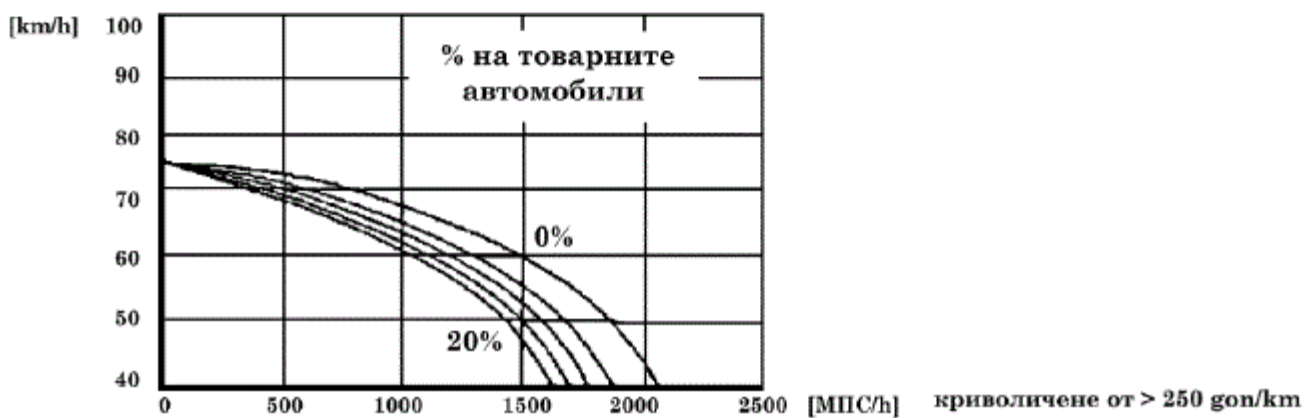
Фигура 11.3. Графики за определяне скоростта на леките автомобили при двулентови пътища
