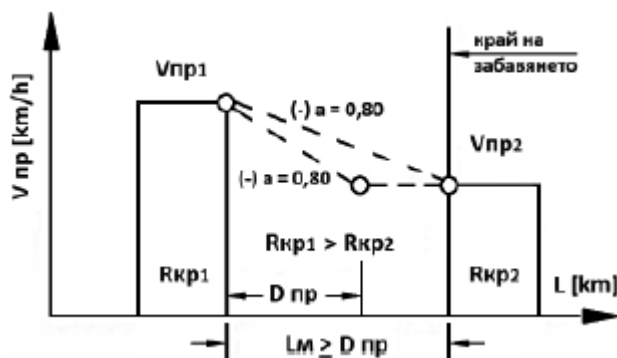
Фигура 1.1. Схема за намаляване на скоростта
