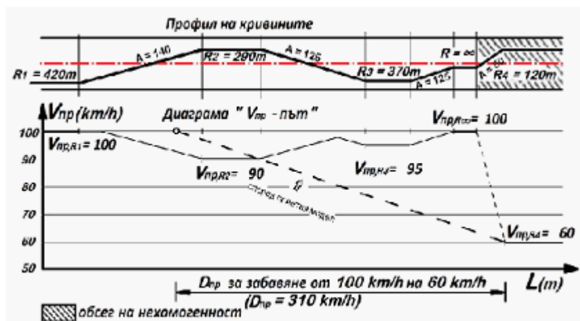
Фигура 1.5. Примерна диаграма "скорост - път"
