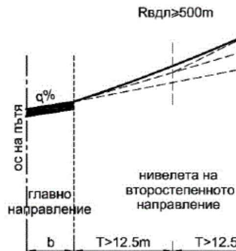
Фигура 46. Присъединяване на второстепенното към главното направление в
