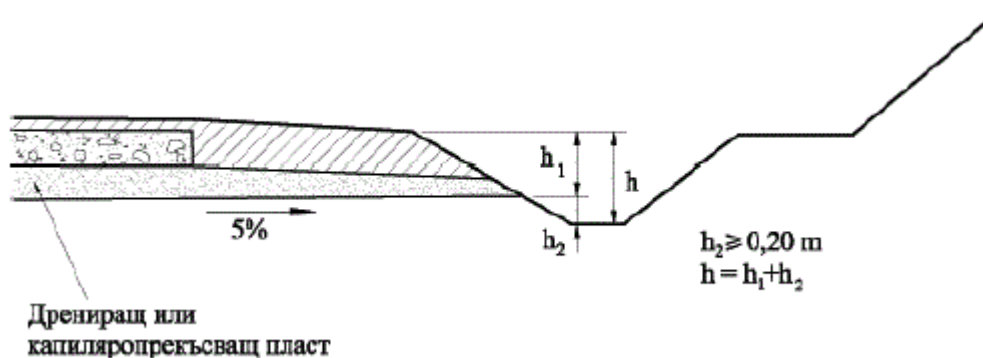
Фигура 108. Определяне на дълбочината на пътния окоп
