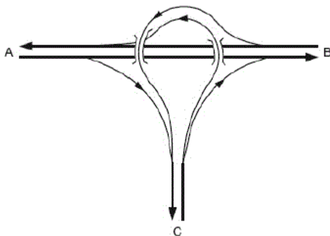
Фигура 76. Пътен възел тип "Круша"
