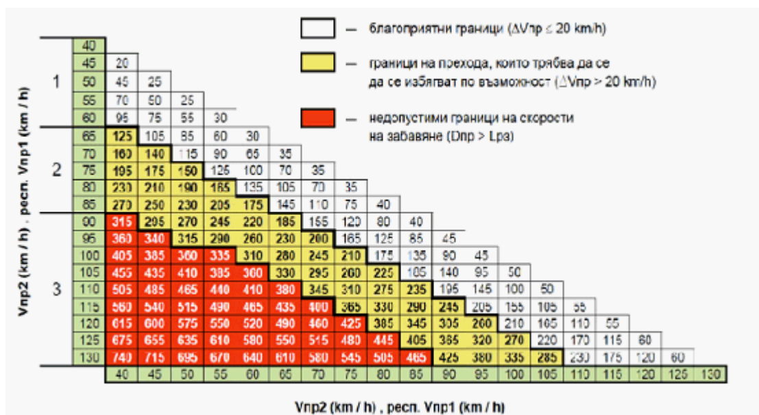
Фигура 1.3. Таблица за определяне на преходния участък D_{np}
