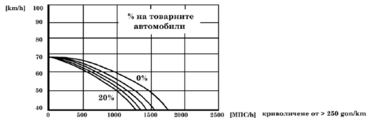
Фигура 11.6. Графики за определяне скоростта на леките автомобили при двулентови пътища
