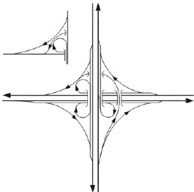
Фигура 67. Модифицирана "Детелина" с полудиректна връзка
