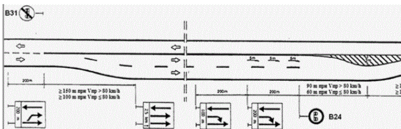
Фигура 12.4. Разположение и примерна сигнализация на допълнителна лента при двулентови пътища
