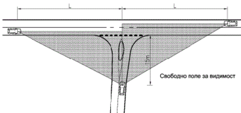
Фигура 42.б. Поле за видимост при приближаване
