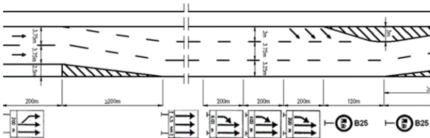
Фигура 12.3. Разположение и примерна сигнализация на допълнителна лента при съществуващи автомагистрали
