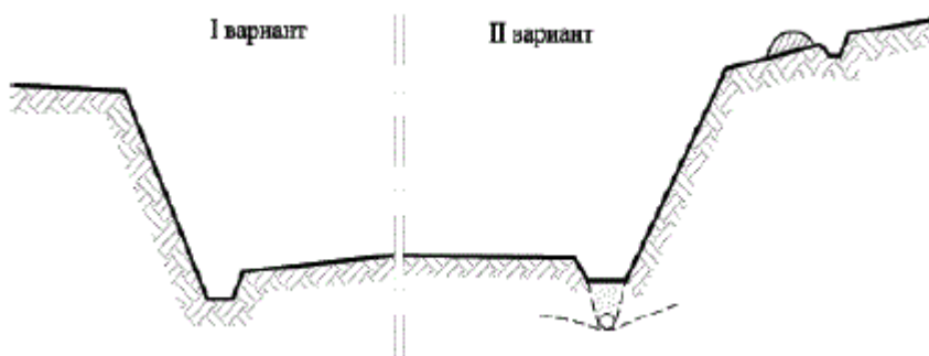
Фигура 143. Схема на отводняване при готов траншеев изкоп
