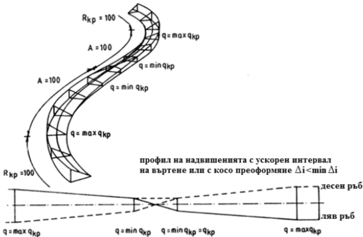
Фигура 8.3. Преоформяне с косо било при дълъг обхват на преоформяне и малък допълнителен наклон \Delta i < \Delta i_{\min}
