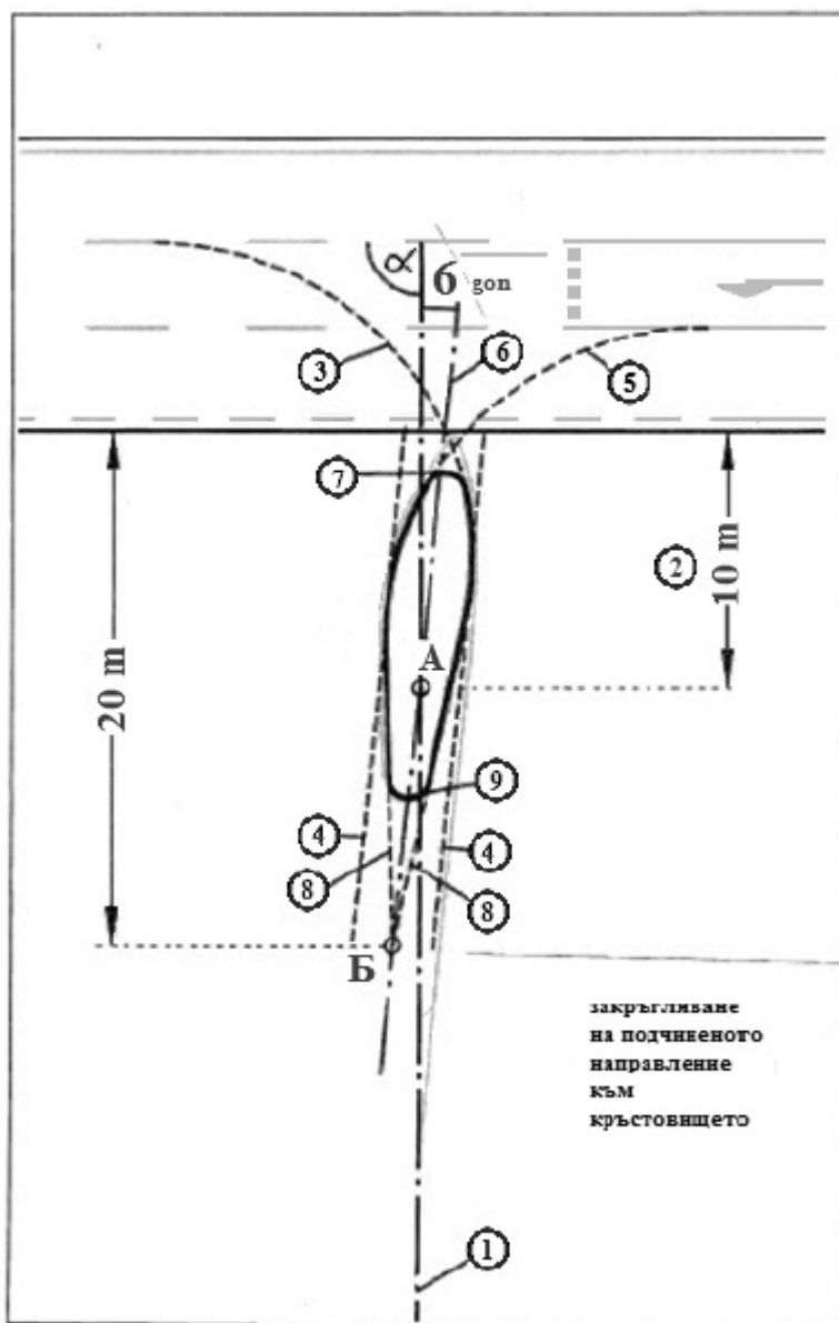
Фигура 13.1. Конструирание на малка капка при ъгъл на пресичане \alpha = 80 \div 120 \text{ gon}
