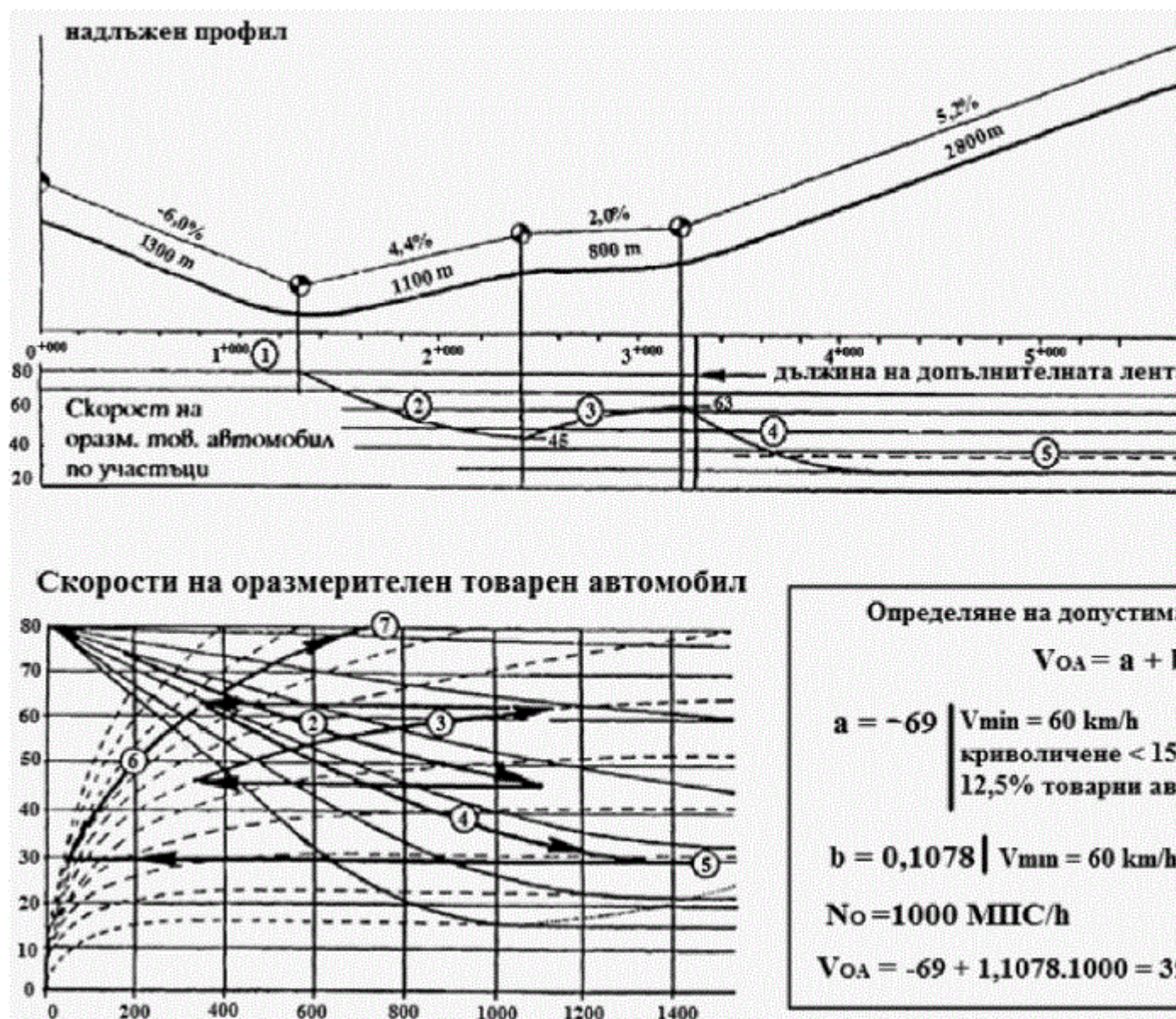
Фигура 12.7. График на скоростта на ОТА
