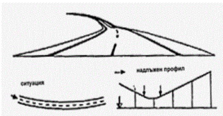
Фигура 16. Оптическо издуване
