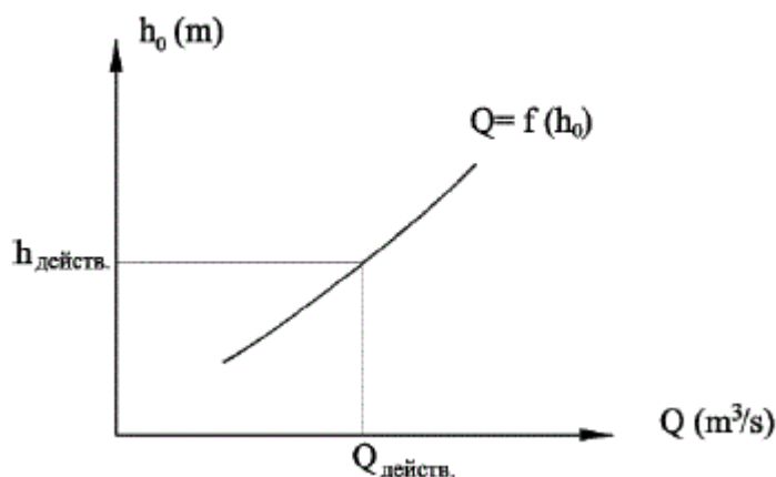
Фигура 110. Графика за определяне на дълбочината на водния поток в пътният окоп
