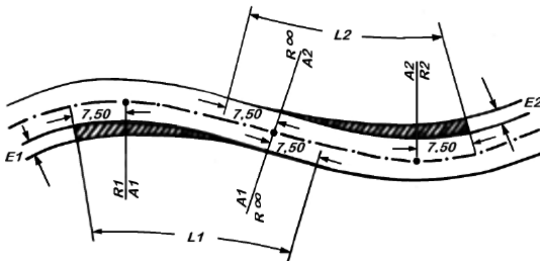
Фигура 7.4. Уширение на настилка при инфлексна клотоида
