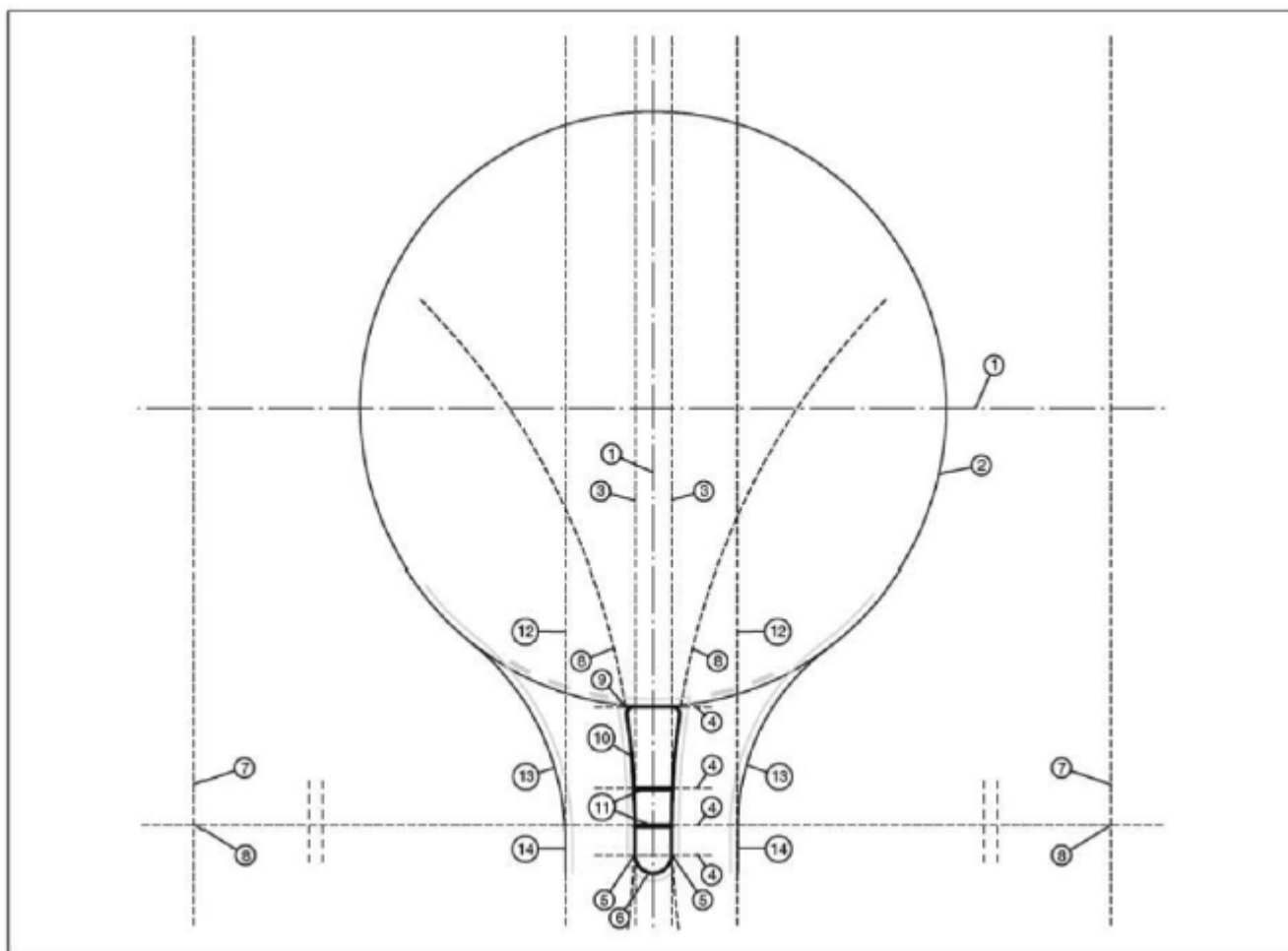
Фигура 14.1. Конструирание на разделител при кръгово кръстовище
