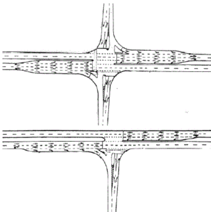
Фигура 49. Кръстовища от III тип
