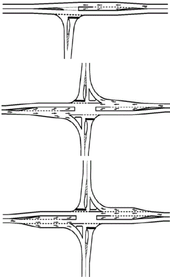
Фигура 48. Кръстовища от II тип
