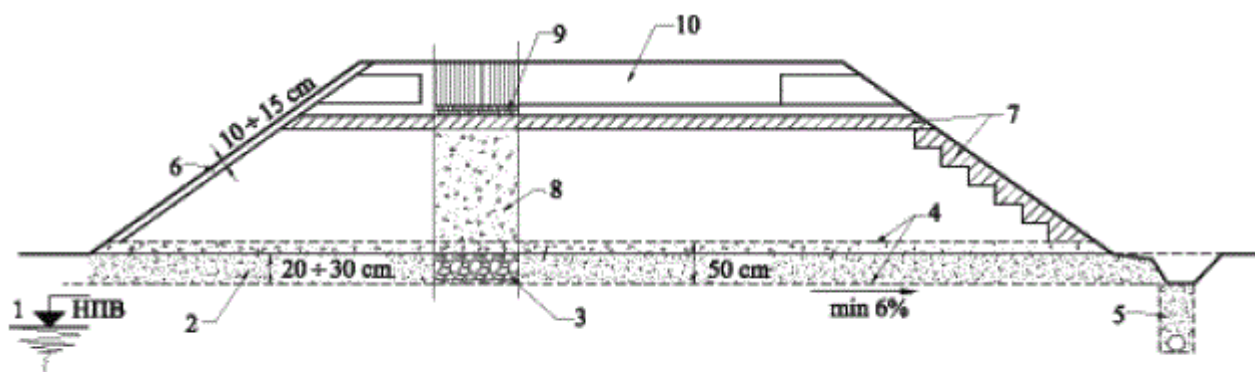
Фигура 119. Система от дренажна възглавница и дренажни пилоти
