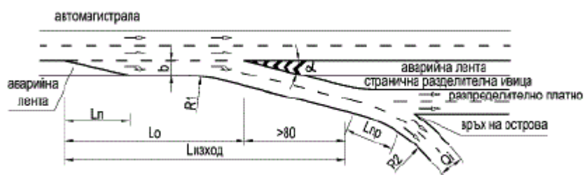
Фигура 93. Изход при разпределително платно
