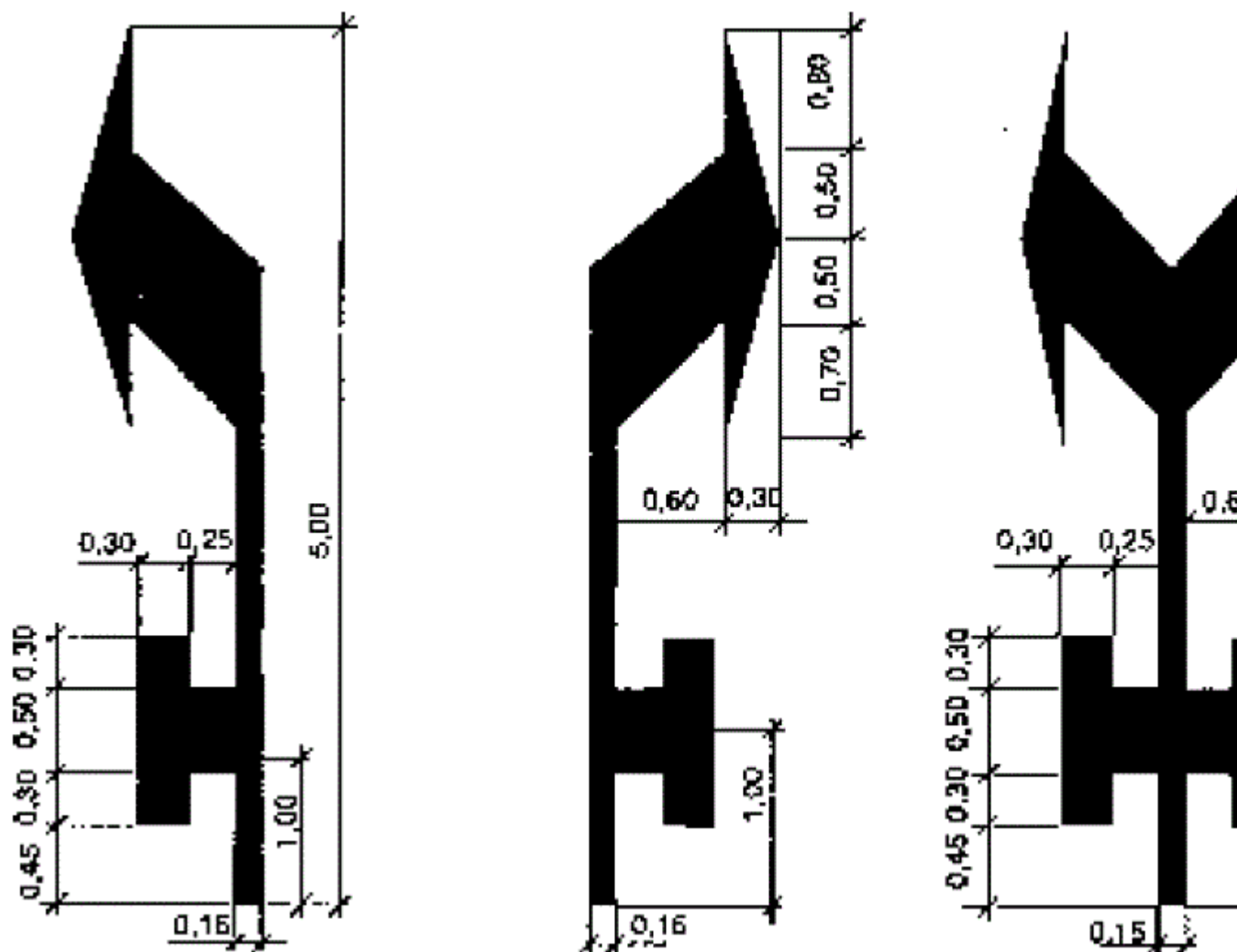
Размери на стрелките при допустима максимална скорост на движение V \leq 50 km/h
