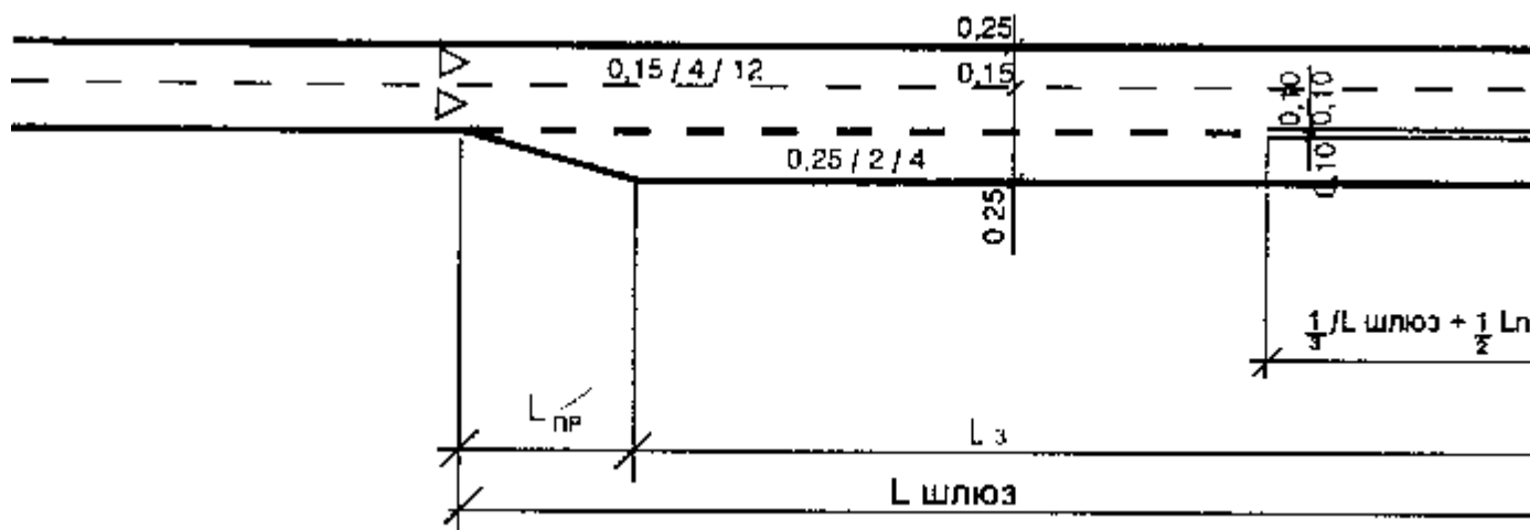
а) лента за забавяне на движението
