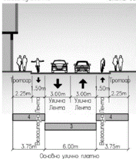
Схема 35
