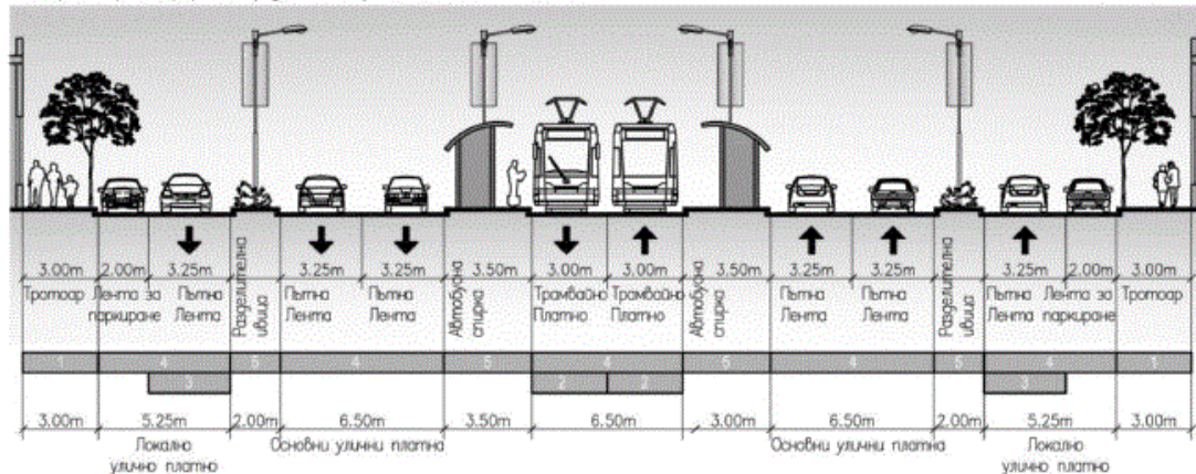
Типизиран напречен профил на градоца магистрала II клас с локални платна
