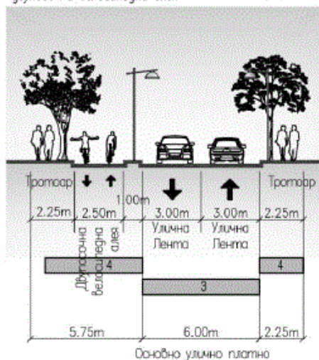
Схема 34
