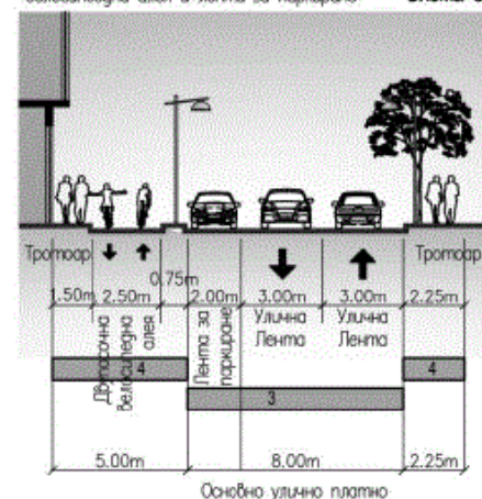
Типизиран напречен профил на обслужваща улица VI клас с велосипедна алея и лента за паркиране Схема 32
