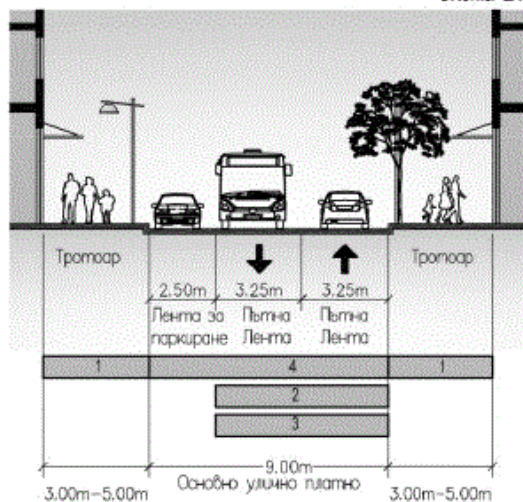
Схема 21
