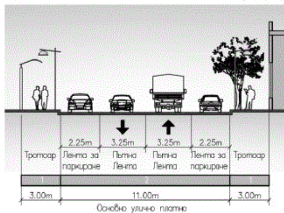
Схема 19
