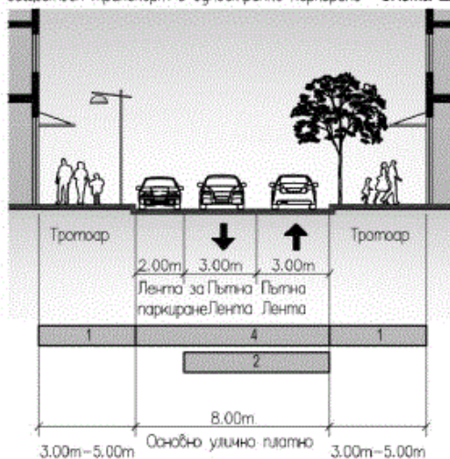
Схема 22
