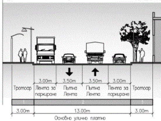
Типизиран напречен профил на главна улица IV клас с двустранно паркиране в индустриална зона
