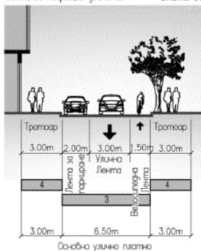
Схема 36
