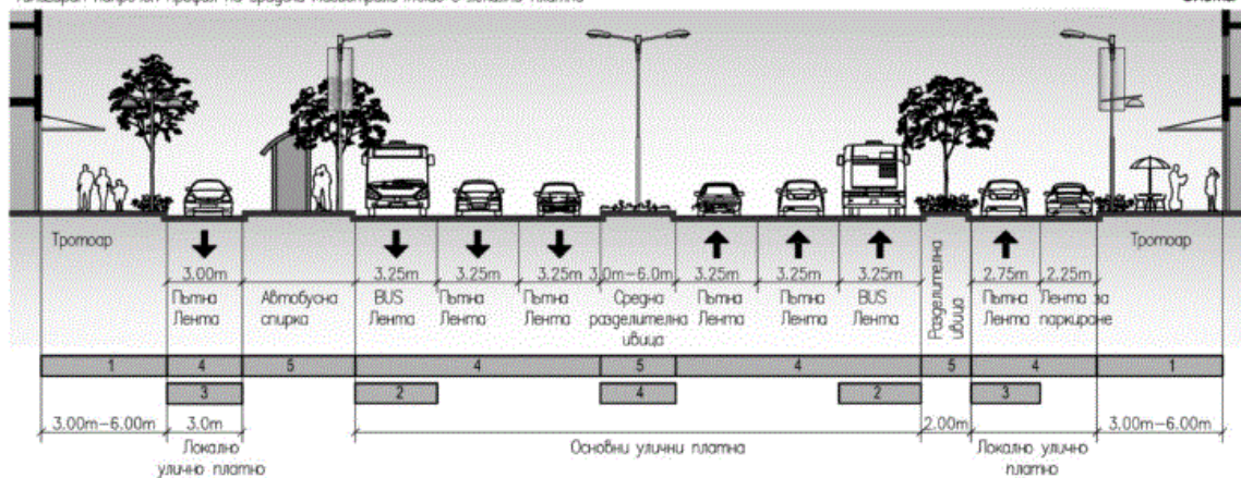
Схема 7
