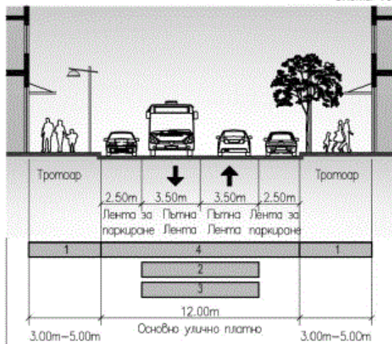
Типизиран напречен профил на главна улица IV клас с обществен транспорт и двустранно паркиране
