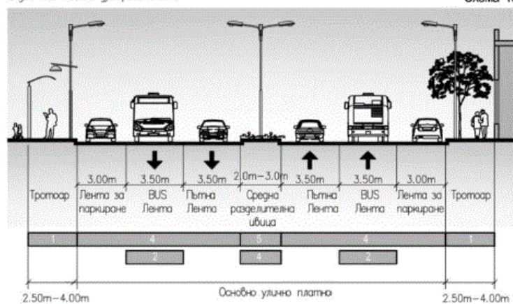
Типизиран напречен профил на районна артерия III клас с две платна в индустриална зона
