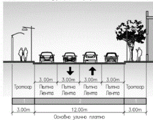
Схема 14
