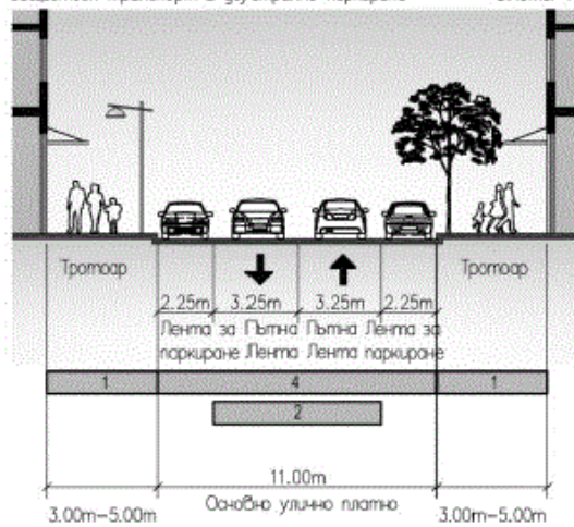
Схема 16
